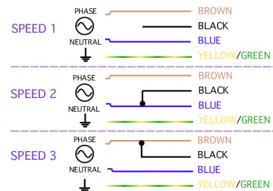
4 WIRE
