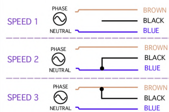
3 WIRE
